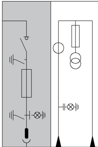
ŞEKİL - 2b AKIM-GERİLİM ÖLÇÜ FONKSİYONEL BİRİMİ
