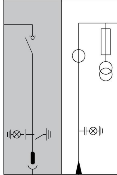
ŞEKİL - 2a AKIM-GERİLİM ÖLÇÜ FONKSİYONEL BİRİMİ
